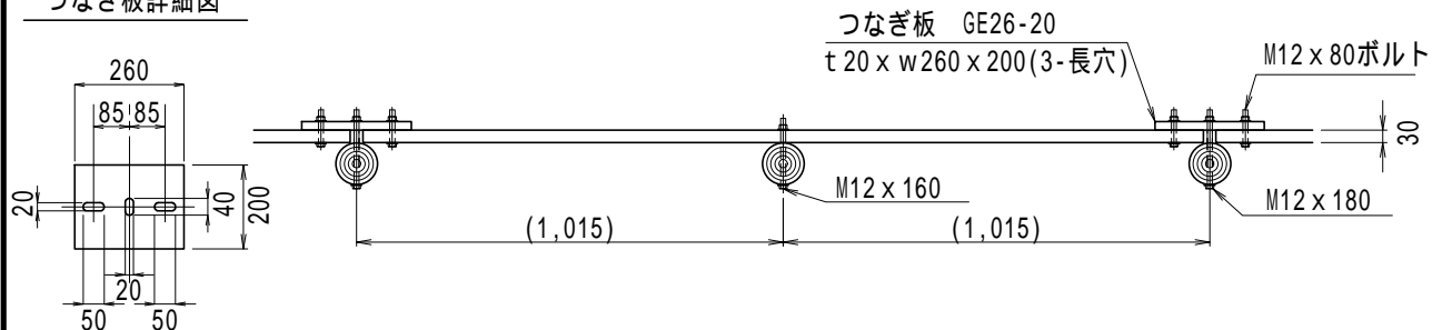
つなぎ板詳細図
