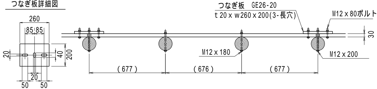
つなぎ板詳細図
